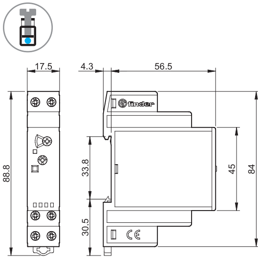
15.10 Conexão a parafuso
