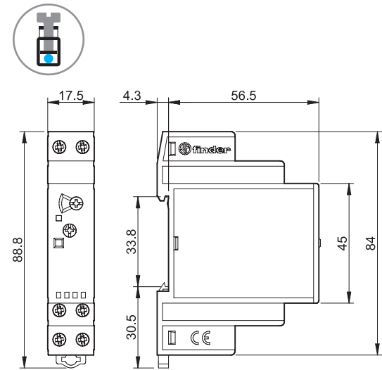
15.11 Conexão a parafuso
